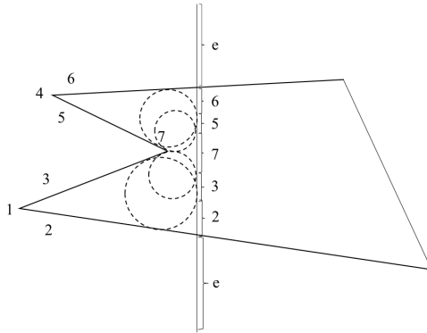
Рис.1 Статус заметающей прямой
