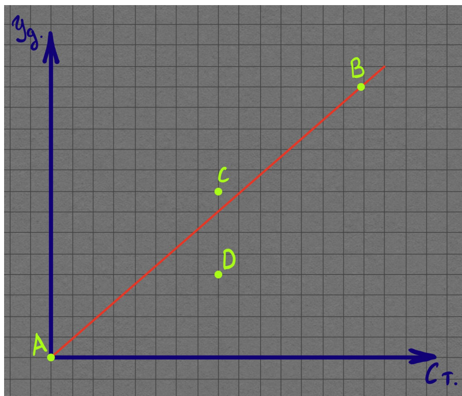
Рис. 1. Принцип Мура
